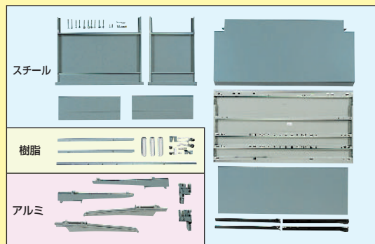
平机ASX-127Hの分解
