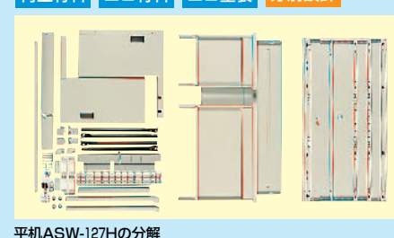
平机ASW-127Hの分解
