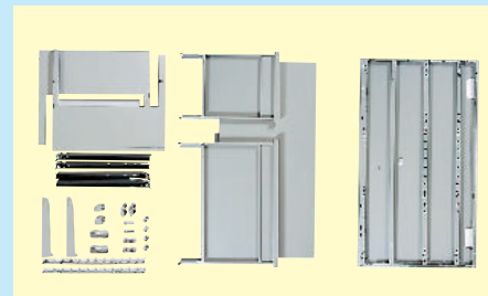
平机CS-127Hの分解
